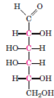
D-Galactose
